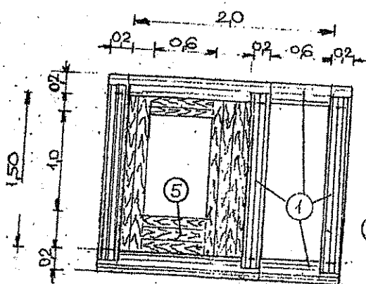
Kétosztályos akna (soros keretézéssel)
