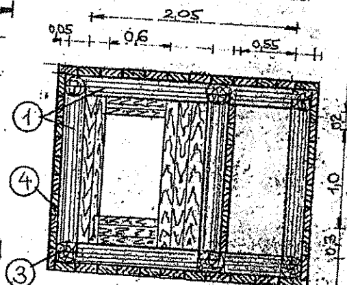
(feszkes keretézéssel, béleléssel)
