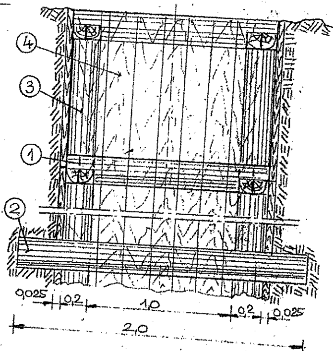
1 sz. melléklet F/Z Kutatbakna (feszkes keretézéssel, béleléssel)
