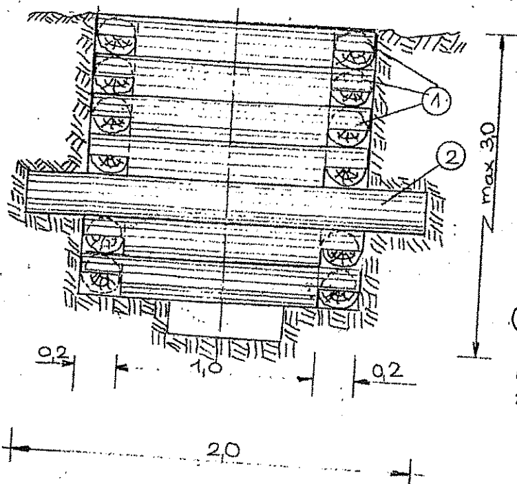
Kétosztályos akna (soros keretézéssel)
